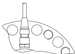
Kabelanschluß gerade
